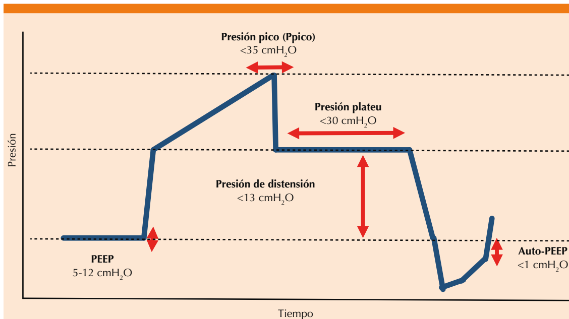
Figura 2. Presiones de vía aérea monitoreadas en la ventilación mecánica de pacientes con COVID-19 vista mediante la curva presión tiempo.
