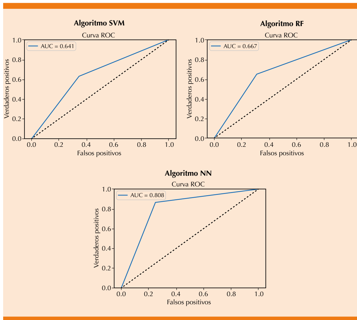
Figura 1. Desempeño de los algoritmos luego del adiestramiento y su puntaje AUC.
